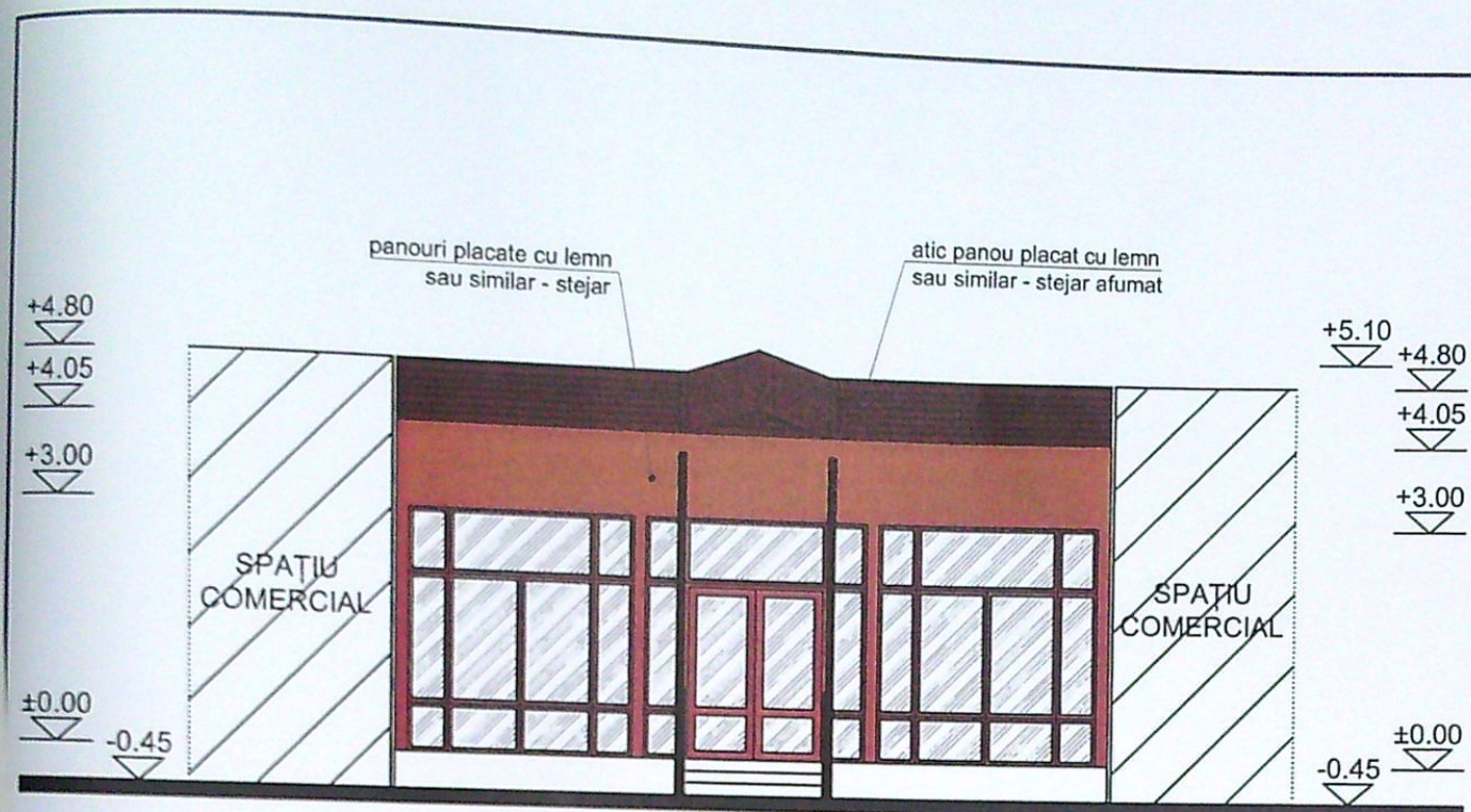
FAȚADA NORD
