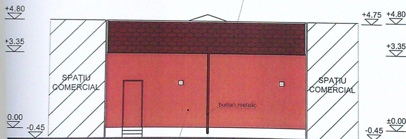
FAȚADA SUD
